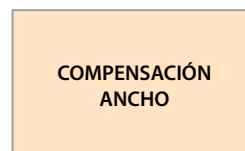
COMPENSACIÓN ANCHO Entre paredes -30/+20 Frontal con lateral -15/+30 Lateral -15+10
