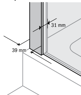
En Hoja de bañera
