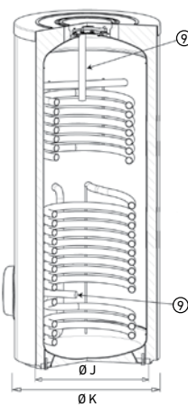
FST 200/500-2E
