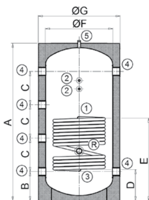
ASA 800-1, 1000-1 y 1500-1
