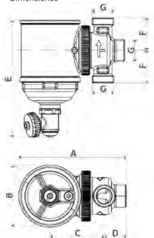
Dimensiones
