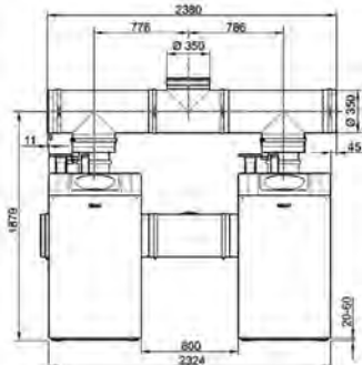
SGB 400 - 610
