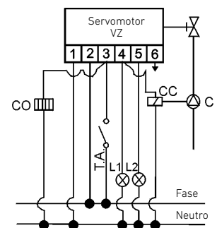
Conexiones eléctricas
