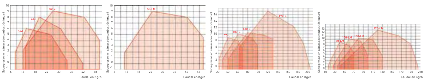
Curvas de caudal presión
