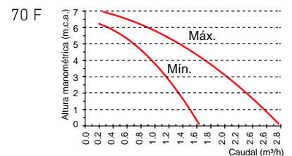
Presión disponible a la salida de la caldera de los circuladores opcionales
