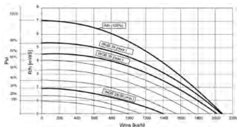
WGB 28 y 38
