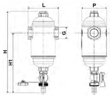
Dimensiones
