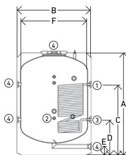
ASA 2000-1, 2500-1, 3000-1, 3500-1, 4000-1 y 5000-1
